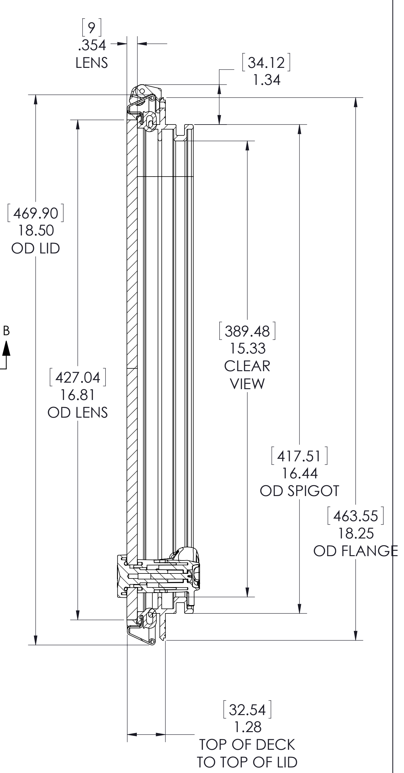
SECTION A-A
